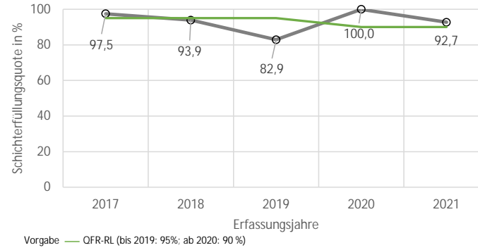
Entwicklung Schichtfüllungsquote Rotkreuzklinikum München (771813) und Vorgabe QFR-RL (2017-2021)
